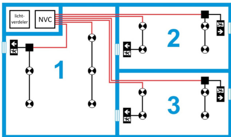
Centrale noodverlichtingsinstallatie zonder onderstations:
