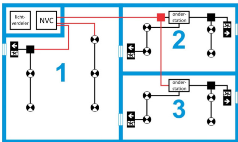
Centrale noodverlichtingsinstallatie met onderstations:
